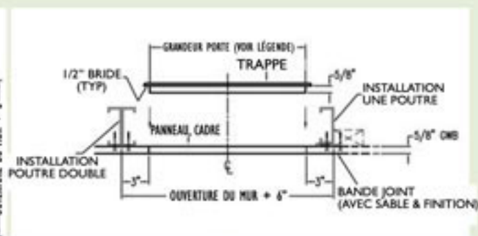
Trappe pour panneau d'accès - Vue de côté (installation de de poutre simple ou double)
